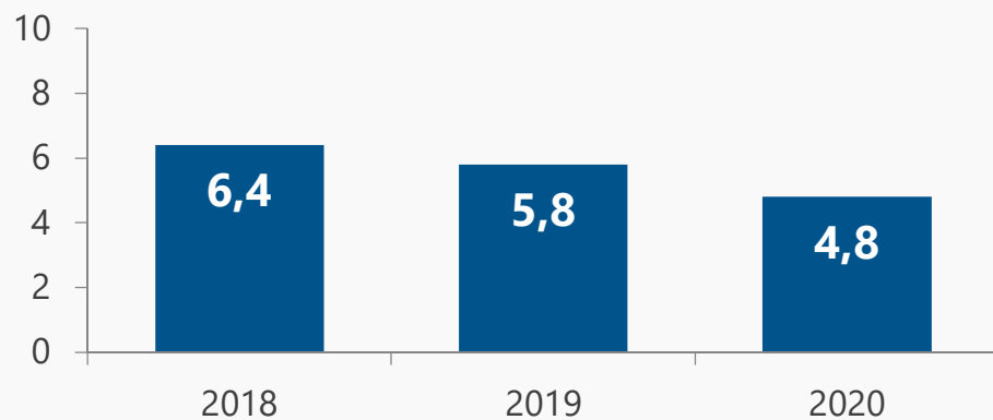
Rapporto clinker/cemento - %
